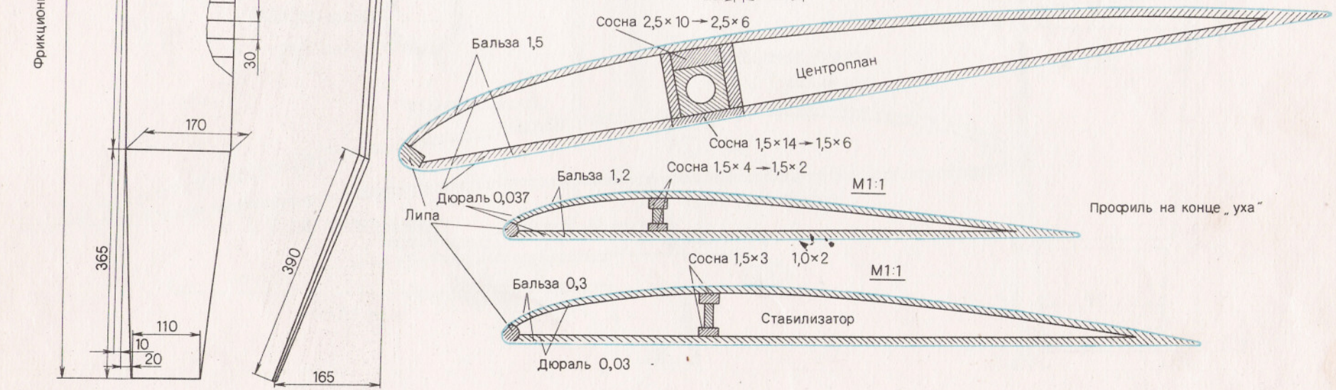
Чертеж модели мастера спорта СССР международного класса, неоднократного чемпиона СССР, призера международных соревнований, члена сборной команды СССР Ю. Абламского (РСФСР).
