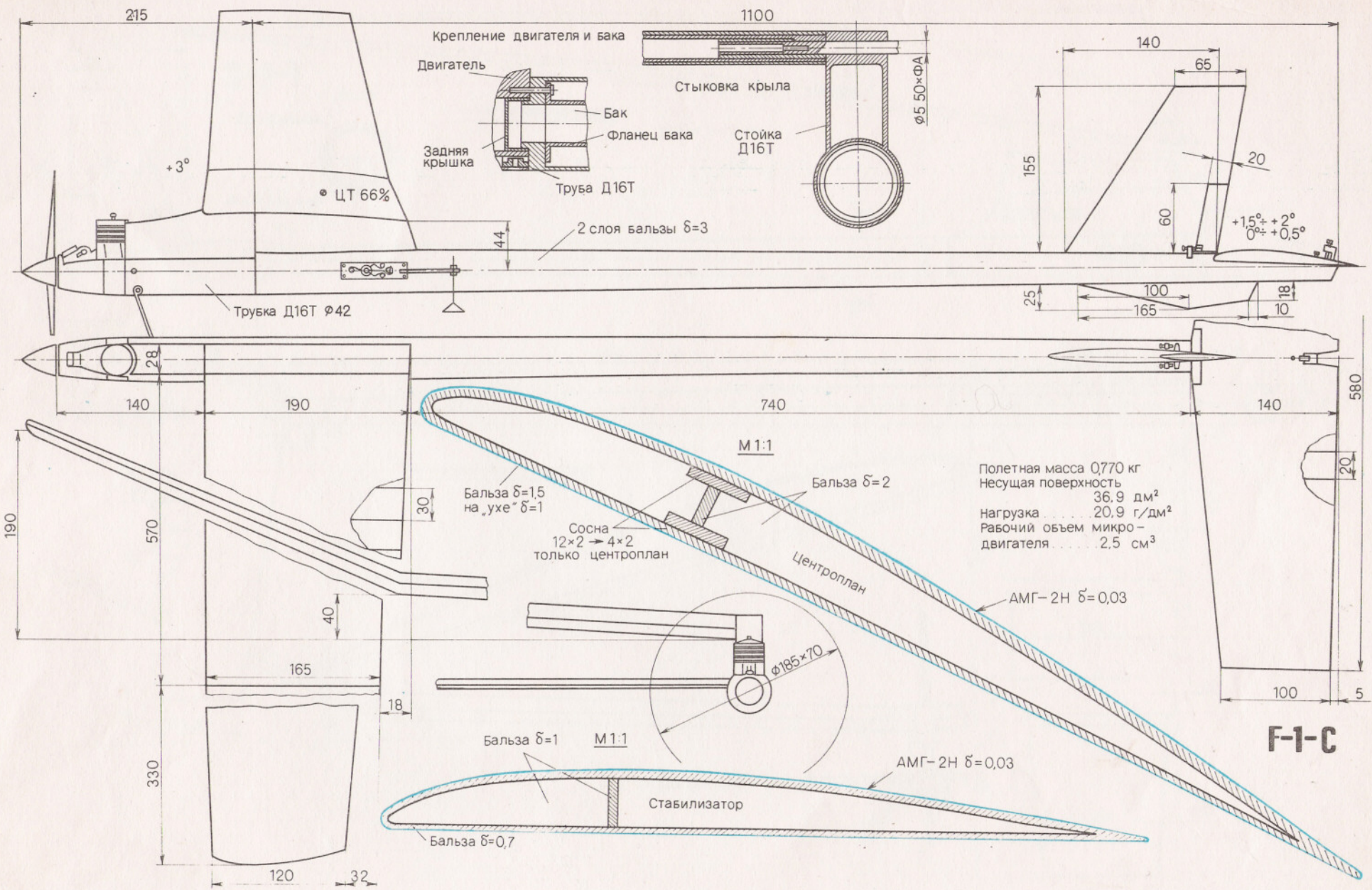
Чертеж модели мастера спорта СССР, призера чемпионата СССР, члена сборной команды РСФСР А. Карпова (РСФСР).
