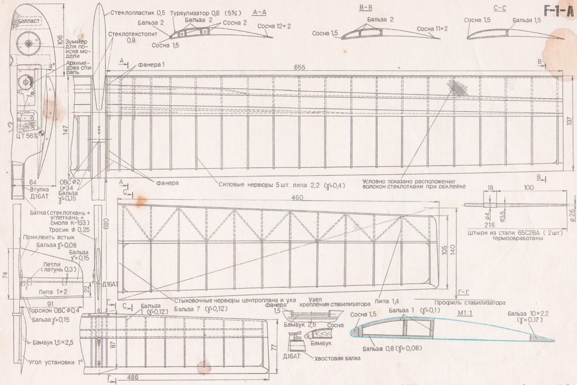
Чертеж модели мастера спорта СССР международного класса, победителя Кубка СССР, призера международных соревнований, члена сборной команды СССР Г. Орлова (г. Москва).
