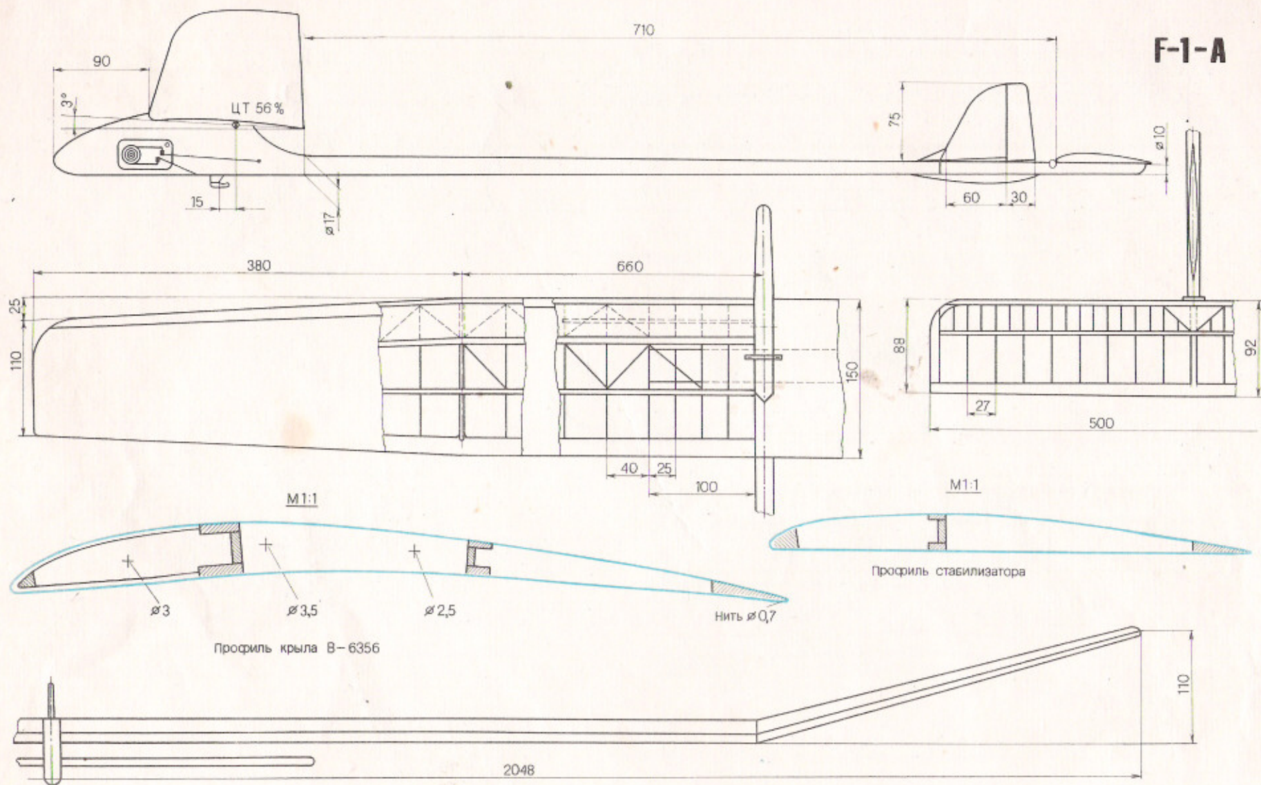
Чертеж модели мастера спорта СССР, призера чемпионата СССР, члена сборной команды СССР В. Стамова (Украина).
