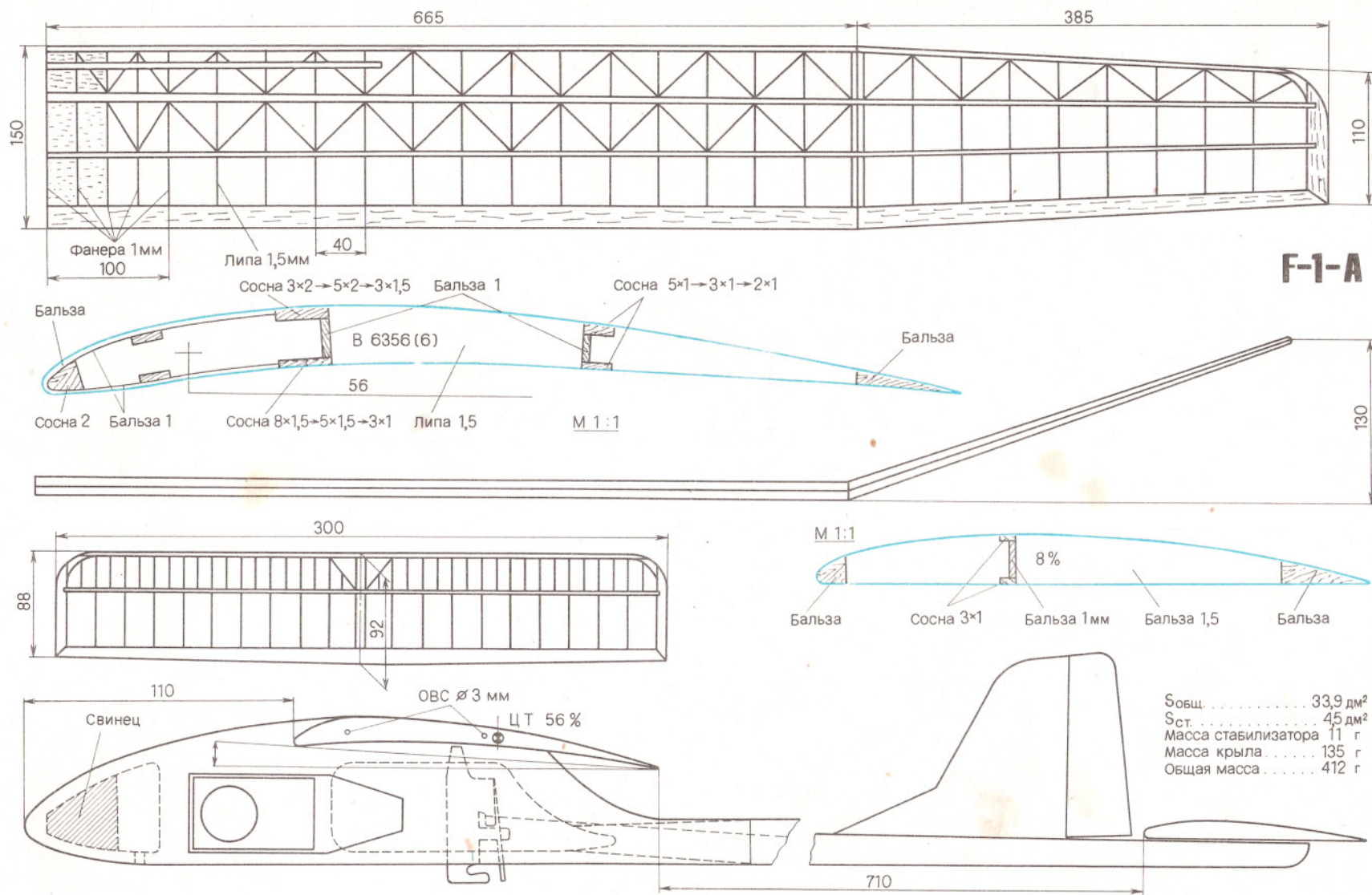
Чертеж модели мастера спорта СССР международного класса, чемпиона мира, члена сборной команды СССР В. Чопа (Украина).
